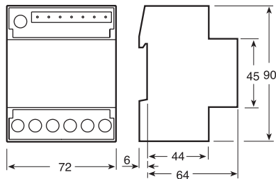
DRM-80-3P
