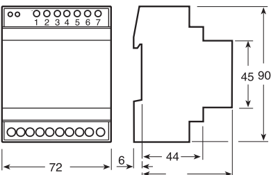
DRM-125-3P
