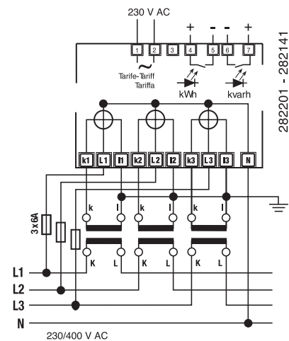
DRM-5-3P
